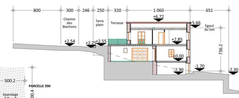
Coupe générale (projet 200e)
